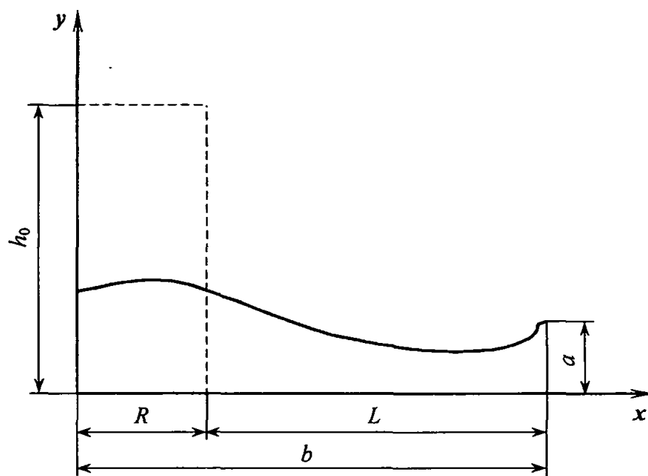
Рис. ПЗ.2. Типичная картина движения жидкости в обваловании при квазимгновенном разрушении резервуара ----- - уровень начального столба жидкости; ——— - уровень жидкости в промежуточный момент времени (результаты расчета)
